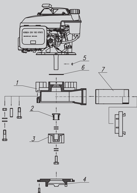
Rysunek techniczny
